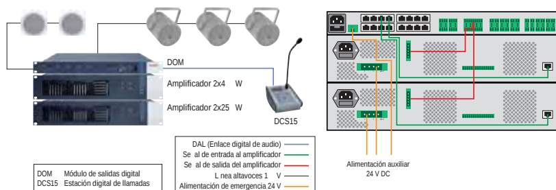
Diagrama general / Amplificadores de potencia 2XD250 y 2XD400 conectados a DOM 4-24
