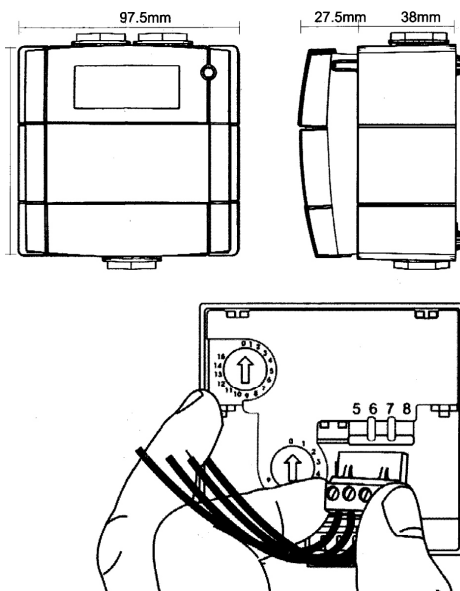
PULSANTI Schemi Di Collegamento
