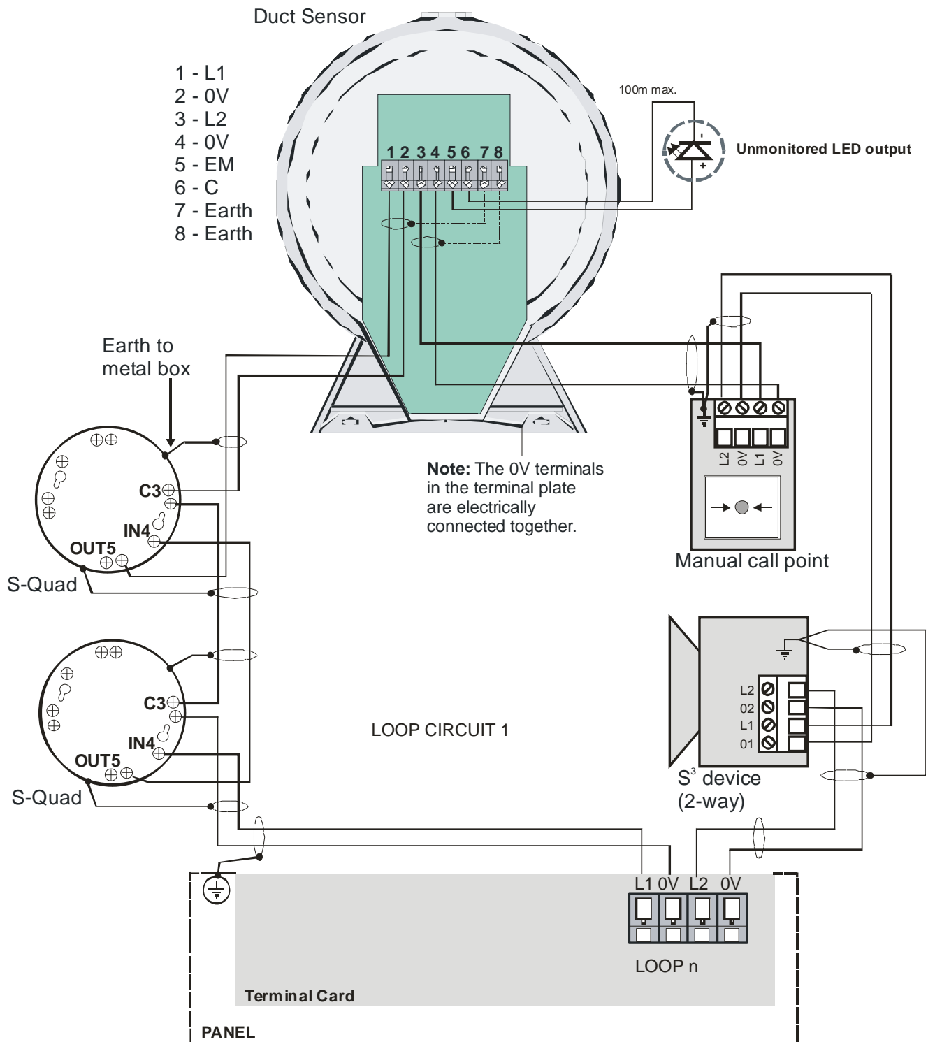
Fig. 25: Loop Wiring
